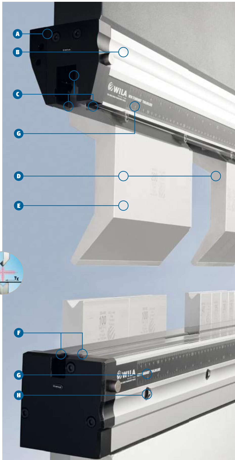
Oberwerkzeug-Halter mit hydraulischen Klemmsystem (HC), pneumatischen Klemmsystem (SL) oder manuellem Klemmsystem (MC).
