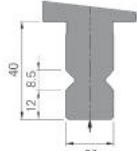
NS III New Standard II Aufnahme
