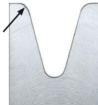
V-Nut mit angewendetem Nitrid-Prozess der Konkurrenz.
