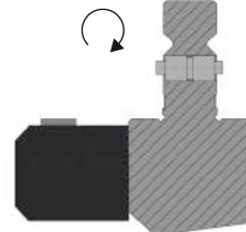
Zusätzliches E2M® Stützlager Lager für große Geißfußwerkzeuge (NS I + II)
