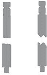
Z-Biegewerkzeuge
